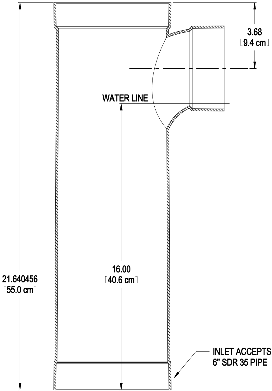
SECTION A-A
